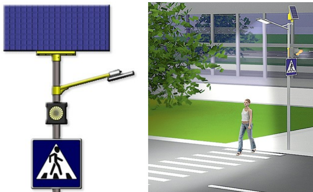
Рисунок 12 Комплект освещения пешеходного перехода на солнечных электростанциях
